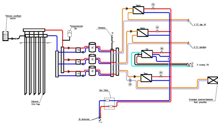
Схема тепло/холодоснабжения здания Прекураторы РБ
