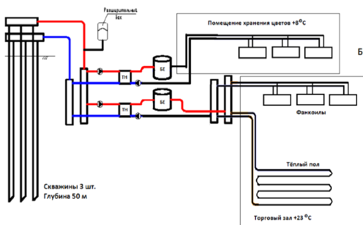
Принципиальная схема тепло-холодо снабжения Павильона "Цветы"
